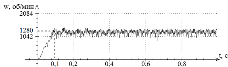
Рисунок 3 – Тахограмма разгона электродвигателя в режиме холостого хода
