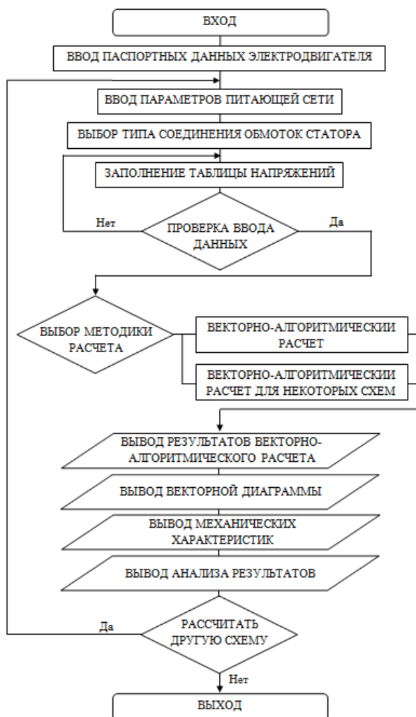
Рисунок 1 – Блок-схема работы программы
