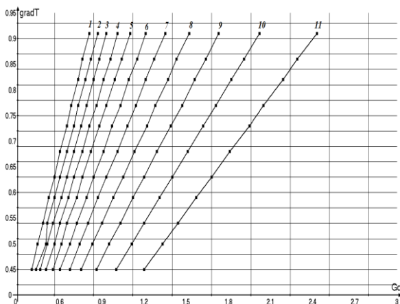
Рисунок 3 - Зависимости G_d=f(\Delta T') при G_A - \text{var} и P_{Э} - \text{var} ., где : 1 - при \Delta T'=15 ; 2 - при \Delta T'=14 ; 3 - при \Delta T'=13 ; 4 - при \Delta T'=12 ; 5 - при \Delta T'=11 ; 6 - при \Delta T'=10 ; 7 - при \Delta T'=9 ; 8 - при \Delta T'=8 ; 9 - при \Delta T'=7 ; 10 - при \Delta T'=6 ; 11 - при \Delta T'=5^{\circ}\text{C}
