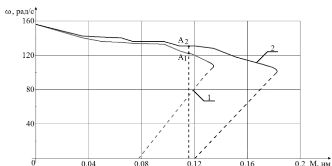
Рисунок 4 – Зависимость скорости от момента на валу:
