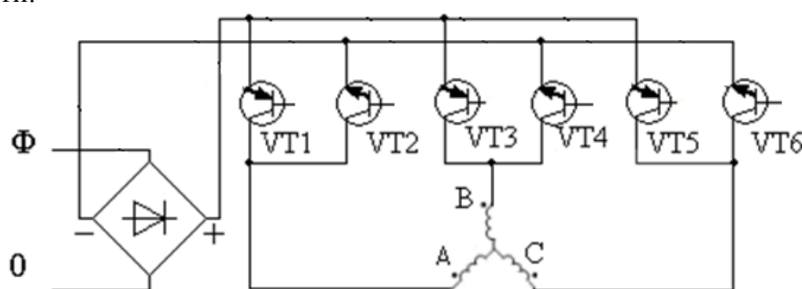
Рисунок 1 - Принципиальная электрическая схема регулируемого транзисторного редуктора трехфазного асинхронного двигателя, питающегося от однофазной сети.
