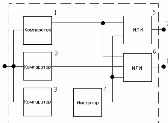
Рисунок 3 – Пороговое устройство с расширенными функциональными возможностями
