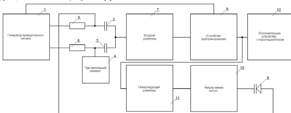
Рисунок 1 – Емкостная адаптивная охранная система
