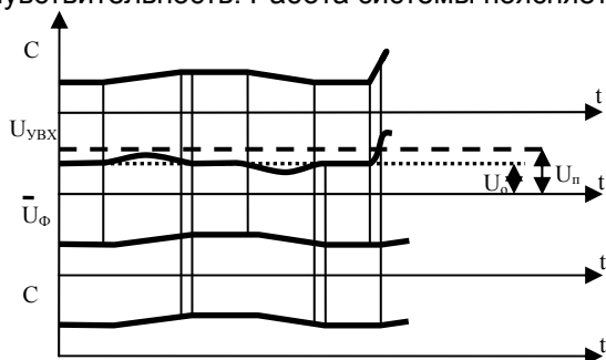
Рисунок 2 – Временные диаграммы работы системы
