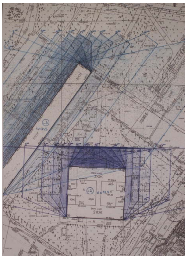
Рисунок 3 – «Конверты теней» для расчета продолжительности инсоляции территории детского сада по ул.Юрина
