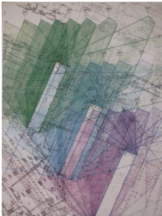
Рисунок 3 – «Конверты теней» для определения инсоляционного режима территории и помещений
